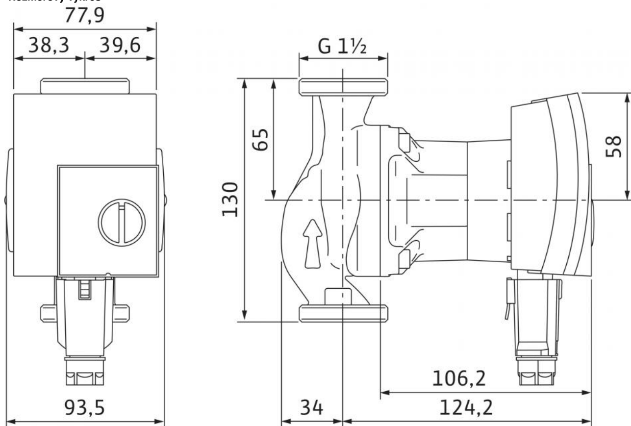
Rozměrový výkres
