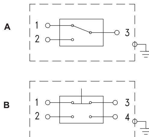
Zapojení spínačů (typ A, B)
