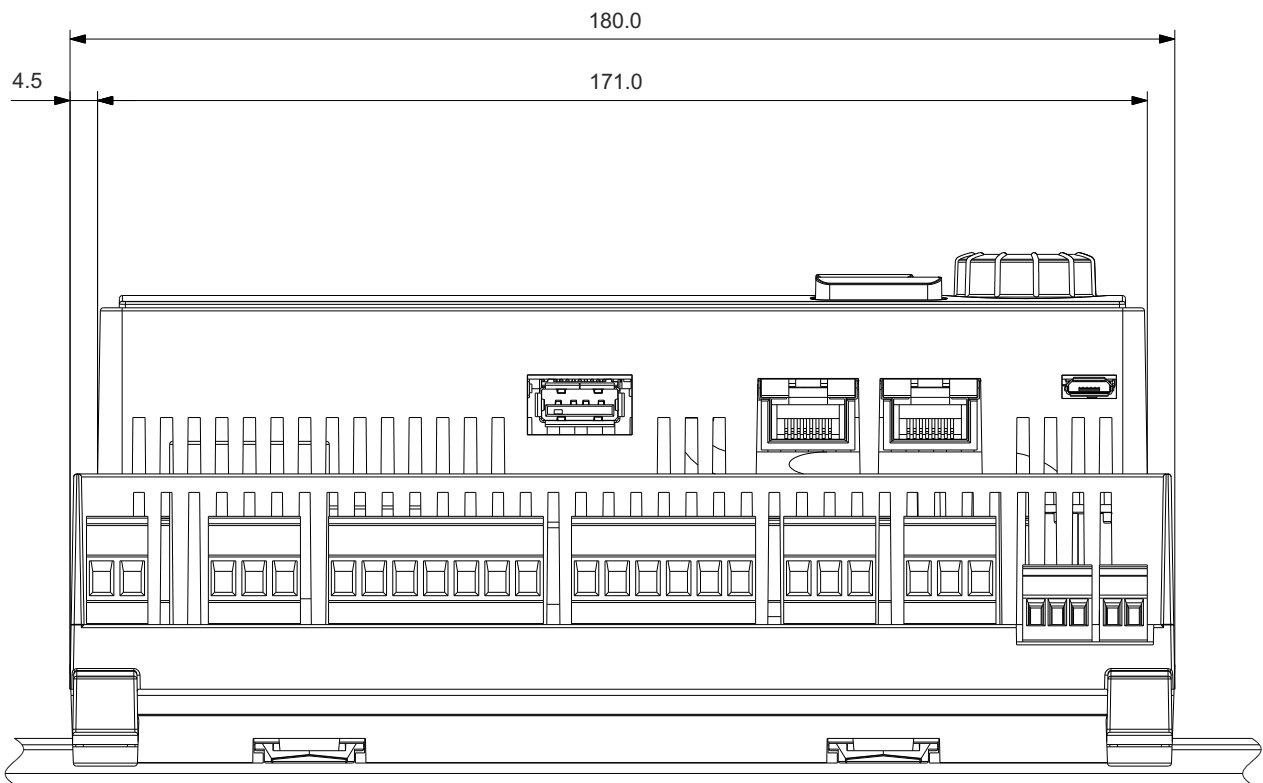
Pohled zdola
